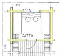
15. Aitta. Lämminala 10,0 m 2 . Terassi 4,5 m 2 .
