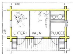
20. Liitteri, vaja ja pucee. Lämminala 14,2 m 2 . Terassi 5,7 m 2 .
