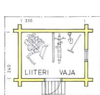
10. Liitteri ja vaja. Lämminala 10,0 m 2 .
