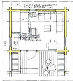
34. Kesämökki. Lämminala 20,3 m 2 . Parvi 3,0 m 2 . Terassi 11,0 m 2 .
