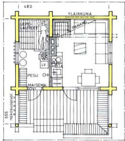
35. Kesämökki, jossa sauna. Lämminala 20,3 m 2 . Pankko 2,1 m 2 . Terassi 12,1 m 2 .
