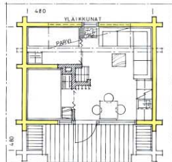
30. Kesämökki. Lämminala 20,3 m 2 . Parvi 3,0 m 2 . Terassi 7,1 m 2 .
