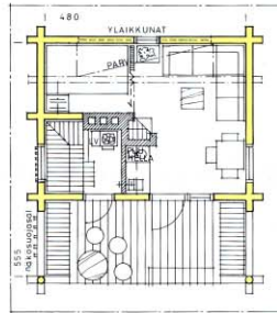
33. Kesämökki, jossa sauna. Lämminala 20,3 m 2 . Parvi 3,0 m 2 . Terassi 10,0 m 2 .
