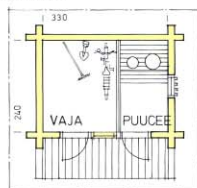
14. Vaja ja pucee. Lämminala 10,0 m 2 . Terassi 4,0 m 2 .
