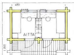
21. Aitta kahdelle. Lämminala 14,2 m 2 . Terassi 6,3 m 2 .
