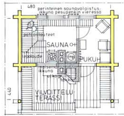
26. Rantasauna, jossa perinteiset patsaslauteet. Lämminala 14,2 m 2 . Terassi 12,0 m 2 .
